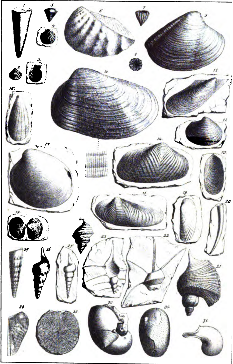
Quenstedt, Jura
